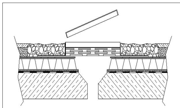
Вариант установки Контрольной шахты
